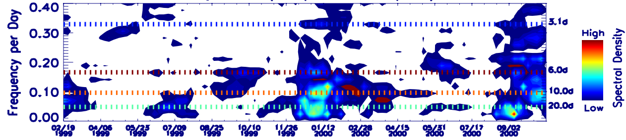
Zonal Wind Spectra (Feb/99 - Oct/00) - 95km
