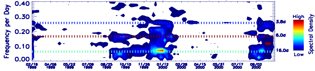
Meridional Wind Spectra (Feb/99 - Oct/00) - 95km
